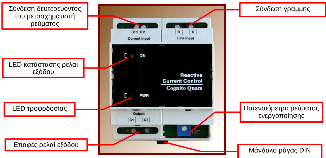
Ελεγκτής αέργου ρεύματος RCC3x
